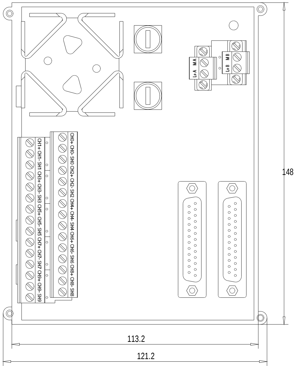
Vorne / Front
