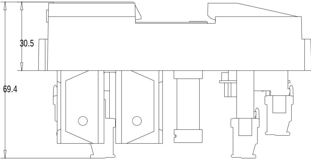
Oben / Top
