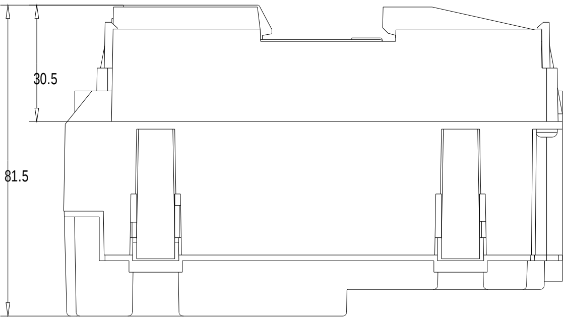
Oben / Top
