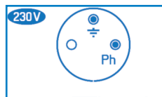
Terre connectée, phase à droite, 230 V.
