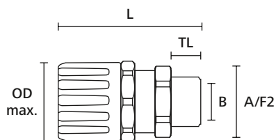
Raccord HelaGuard, droit avec filetage externe tournant
