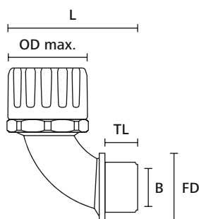
Raccord HelaGuard, coudé à 90° avec filetage externe
