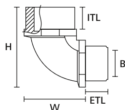
Coupleur coudé à 90° HelaGuard
