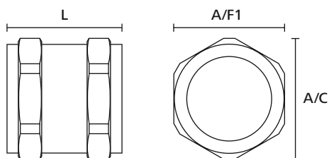
Coupleur fileté HelaGuard
