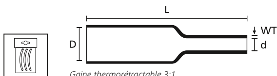
Gaine thermorétractable 3:1
