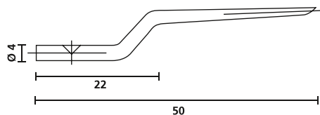
Bec de rechange NA1K/3
