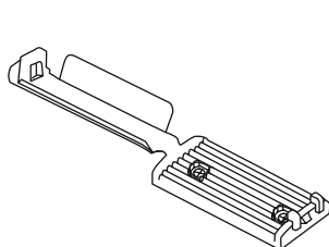
Clip de la série FKH, adhésif ou à visser (à l'aide d'une vis M3)
