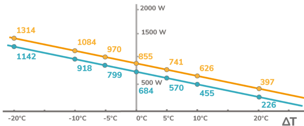
Puissance thermique de la version isolée en Watt en fonction de ( T_{\text{eau}} - T_{\text{air}} ) pour G=800 et G=1000\text{W/m}^2
