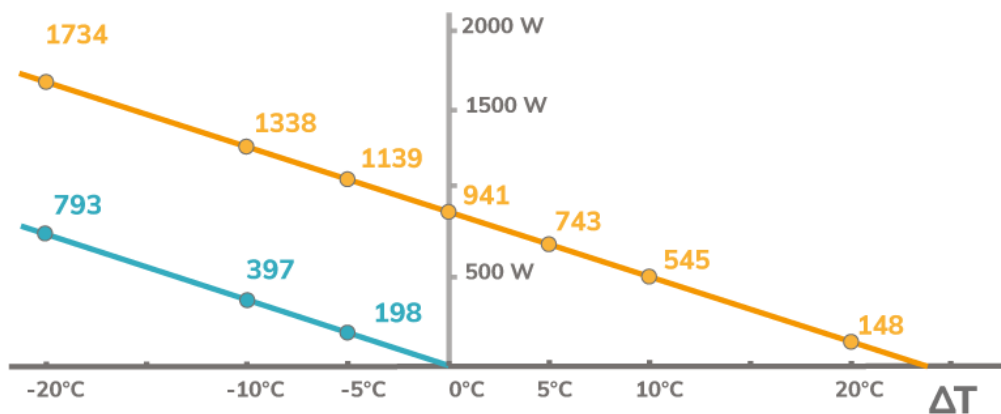
Puissance thermique de la version non isolée en Watt en fonction de ( T_{\text{eau}} - T_{\text{air}} ) pour G=0 et G=1000\text{W/m}^2
