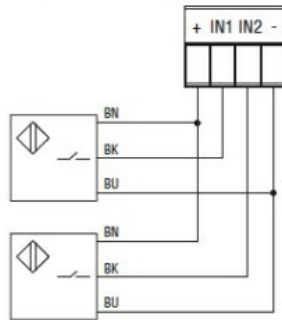
Ingresso da sensori alimentati (vedi note sotto) Supplied sensor inputs (See note below)
