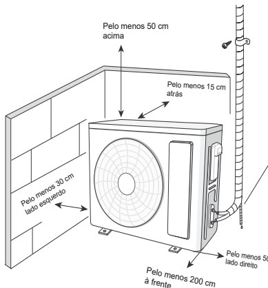
Configuração das ligações frigoríficas
