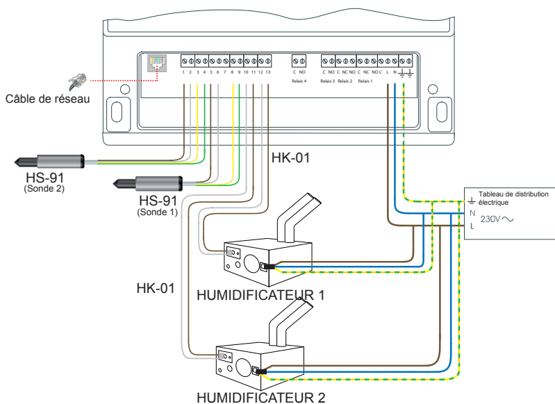
Figure 9. Schéma de raccordement de certains hygrostat.
