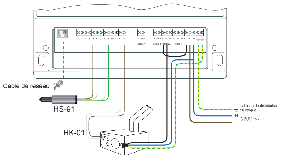
Figure 9. Schéma de raccordement de certains hygrostat.
