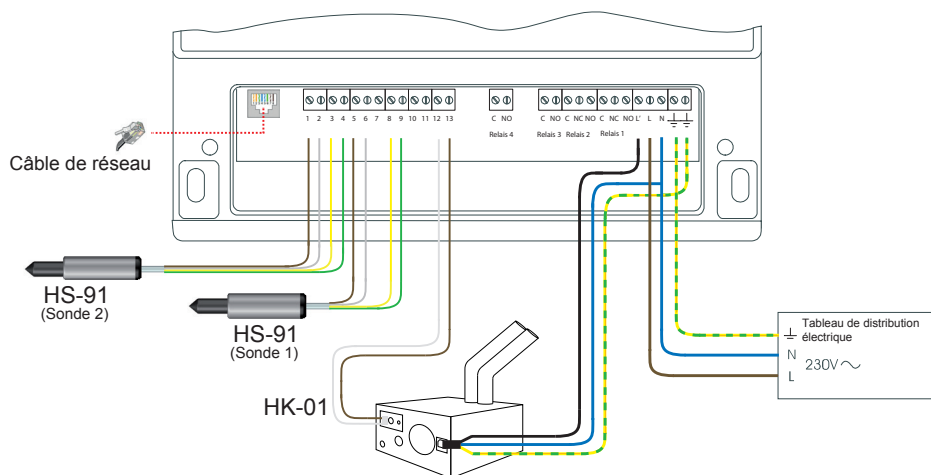
Figure 11. Schéma de raccordement de hygrostat avec contrôle maximal.
