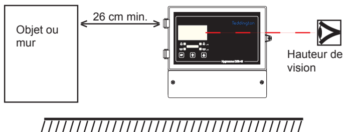
Figure 2. Installation du régulateur
