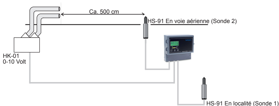
Figure 8. Hygrostat avec contrôle maximal.
