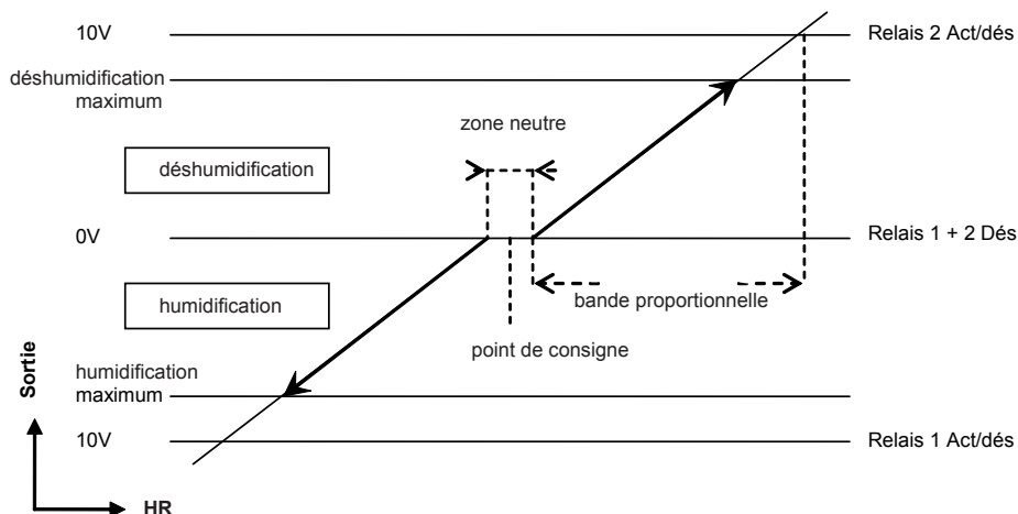
Figure 8. Fonctionnement général de l'hygrostat
