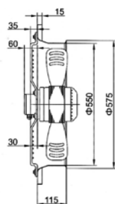
■ TF MASC-B6E-550 MOTO-VENTILATEUR-AXIAL S/ SUPPORT CARRE AVEC HELICE
