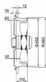
TF MASC-B6D-450 MOTO-VENTILATEUR-AXIAL S/ SUPPORT CARRE AVEC HELICE
