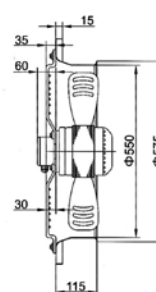
TF MASC-B6D-550 MOTO-VENTILATEUR-AXIAL S/ SUPPORT CARRE AVEC HELICE
