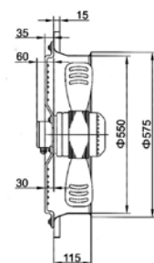
■ TF MASC-B4E-550 MOTO-VENTILATEUR-AXIAL S/ SUPPORT CARRE AVEC HELICE
