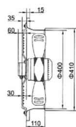
TF MASC-B4D-400 MOTO-VENTILATEUR-AXIAL S/ SUPPORT CARRE AVEC HELICE
