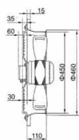
TF MASC-B4E-450 MOTO-VENTILATEUR-AXIAL S/ SUPPORT CARRE AVEC HELICE
