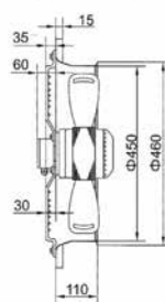
■ TF MASC-B6E-450 MOTO-VENTILATEUR-AXIAL S/ SUPPORT CARRE AVEC HELICE
