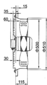
TF MASC-B6D-500 MOTO-VENTILATEUR-AXIAL S/ SUPPORT CARRE AVEC HELICE
