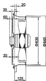
■ TF MASC-B4E-630 MOTO-VENTILATEUR-AXIAL S/ SUPPORT CARRE AVEC HELICE
