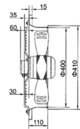
■ TF MASC-B6E-400 MOTO-VENTILATEUR-AXIAL S/ SUPPORT CARRE AVEC HELICE
