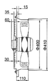
TF MASC-B6D-400 MOTO-VENTILATEUR-AXIAL S/ SUPPORT CARRE AVEC HELICE
