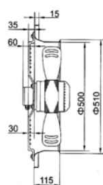
TF MASC-B4D-500 MOTO-VENTILATEUR-AXIAL S/ SUPPORT CARRE AVEC HELICE
