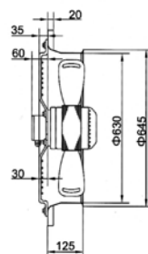
■ TF MASC-B6E-630 MOTO-VENTILATEUR-AXIAL S/ SUPPORT CARRE AVEC HELICE
