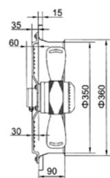
■ TF MASC-B4E-350 MOTO-VENTILATEUR-AXIAL S/ SUPPORT CARRE AVEC HELICE
