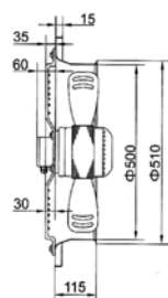
■ TF MASC-B4E-500 MOTO-VENTILATEUR-AXIAL S/ SUPPORT CARRE AVEC HELICE
