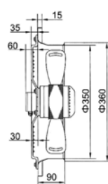
TF MASC-B4D-350 MOTO-VENTILATEUR-AXIAL S/ SUPPORT CARRE AVEC HELICE
