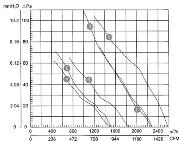
■ COURBE N°2 4E-350 220V/50Hz 0-90Pa (20Pa-1960m 3 /h)
