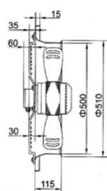
■ TF MASC-B6E-500 MOTO-VENTILATEUR-AXIAL S/ SUPPORT CARRE AVEC HELICE
