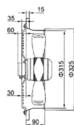
TF MASC-B4D-300 MOTO-VENTILATEUR-AXIAL S/ SUPPORT CARRE AVEC HELICE
