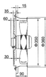
■ TF MASC-B6E-350 MOTO-VENTILATEUR-AXIAL S/ SUPPORT CARRE AVEC HELICE
