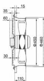
TF MASC-B4D-450 MOTO-VENTILATEUR-AXIAL S/ SUPPORT CARRE AVEC HELICE
