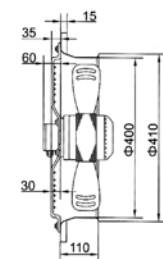
■ TF MASC-B4E-400 MOTO-VENTILATEUR-AXIAL S/ SUPPORT CARRE AVEC HELICE
