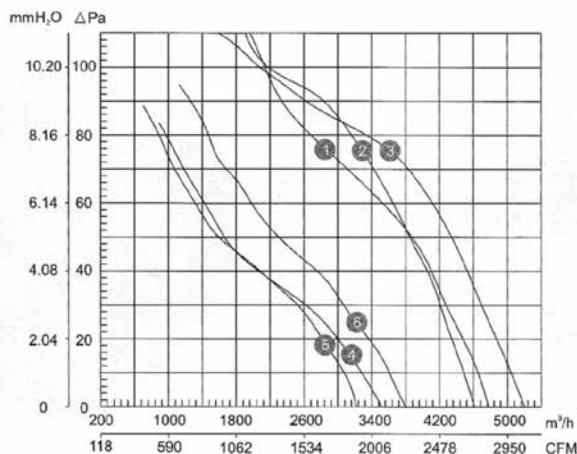
COURBE N°4 6D-450 380V/50Hz 0~90Pa (20Pa-3000m 3 /h)
