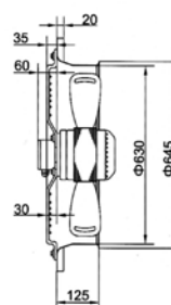
TF MASC-B4D-630 MOTO-VENTILATEUR-AXIAL S/ SUPPORT CARRE AVEC HELICE
