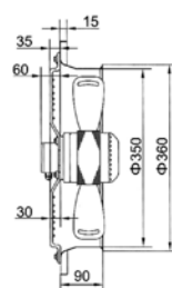
TF MASC-B6D-350 MOTO-VENTILATEUR-AXIAL S/ SUPPORT CARRE AVEC HELICE
