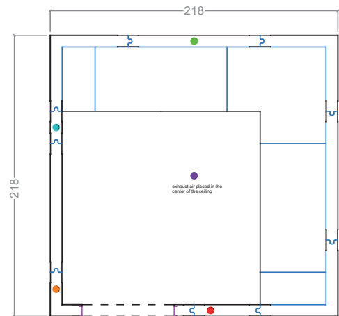
PLAN AVEC PORTE SUR LE CÔTÉ GAUCHE
