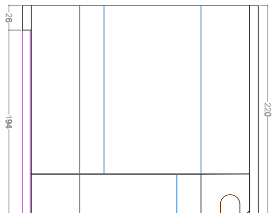
COUPE
