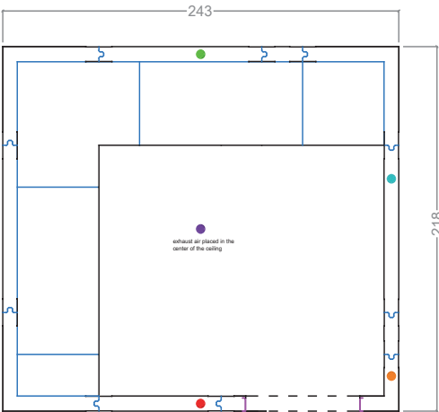
PLAN AVEC PORTE SUR LE CÔTÉ DROIT
