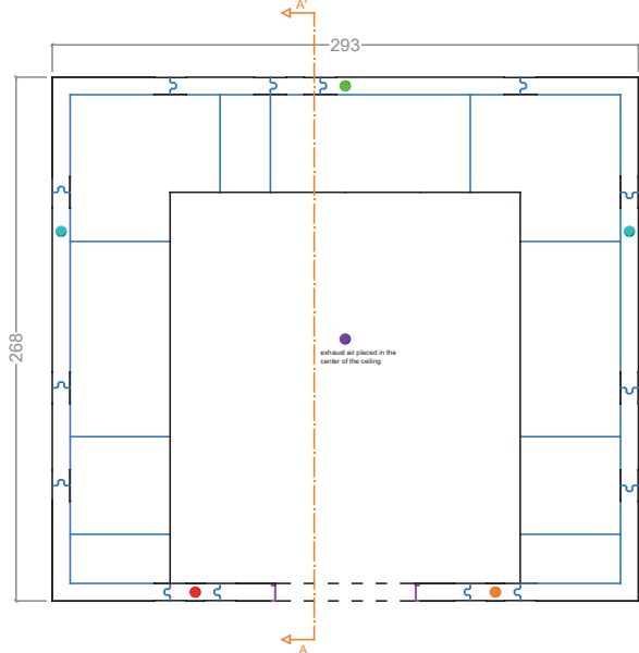
PLAN AVEC PORTE CENTRALE
