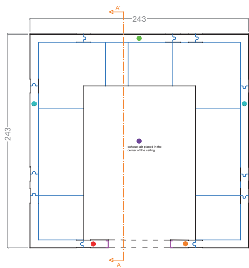
PLAN AVEC PORTE CENTRALE
