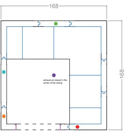
PLAN AVEC PORTE SUR LE CÔTÉ GAUCHE
