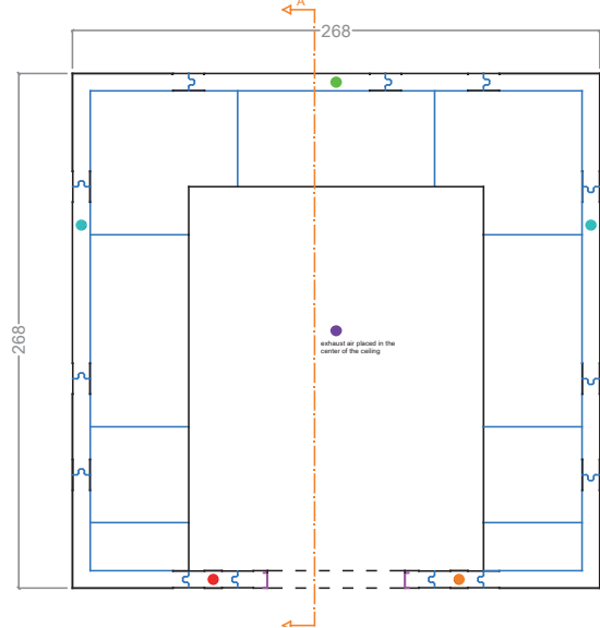
PLAN AVEC PORTE CENTRALE
