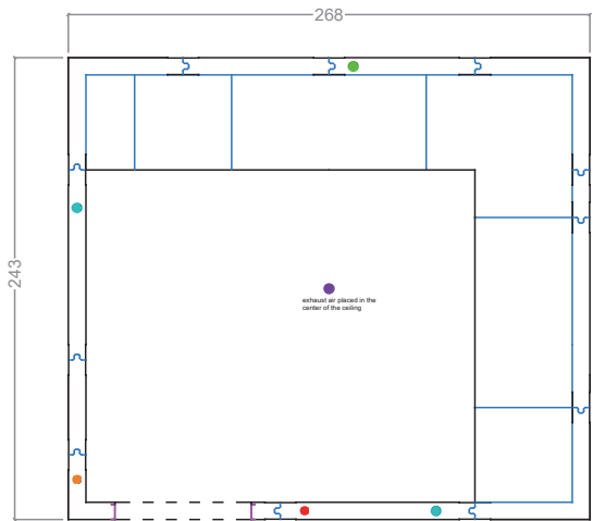
PLAN AVEC PORTE SUR LE CÔTÉ GAUCHE
