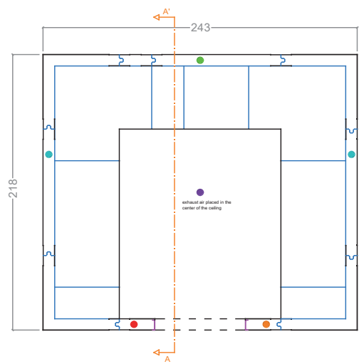
PLAN AVEC PORTE CENTRALE
