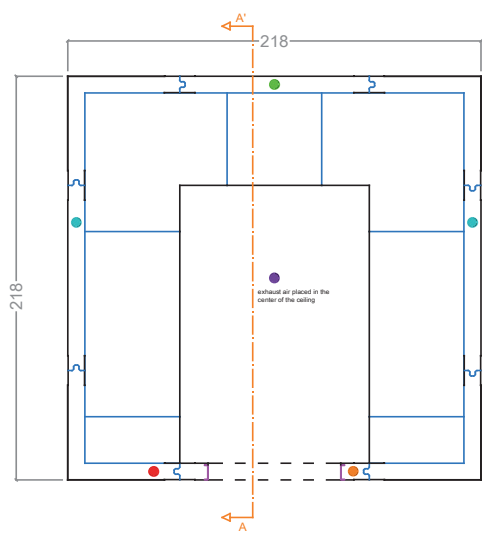
PLAN AVEC PORTE CENTRALE
