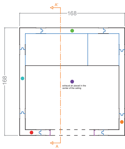
PLAN AVEC PORTE CENTRALE
