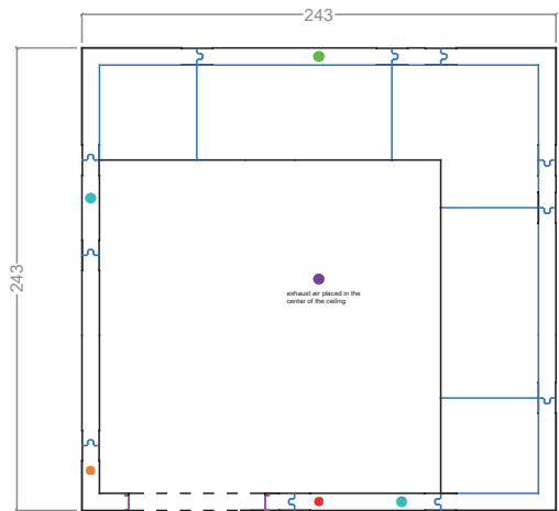
PLAN AVEC PORTE SUR LE CÔTÉ GAUCHE
