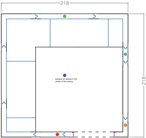
PLAN AVEC PORTE SUR LE CÔTÉ DROIT
