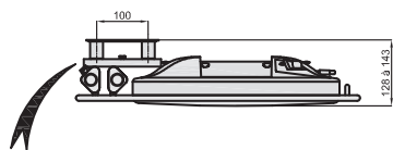
Détail de la fixation / Befestigungsdetail
