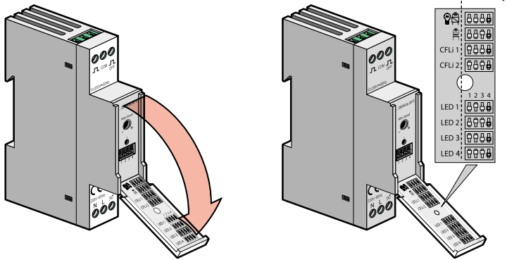
Fig. 3 / Abb. 3 / Obr. 3 Minimumniveau instellen / Paramétrage du niveau minimum / Minimaleistung einstellen / Setting the minimum level / Nastavenie minimálnej úrovne
