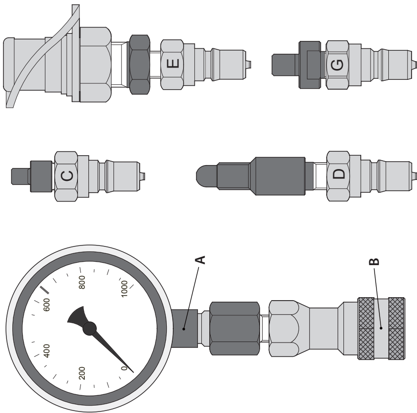
FIG. 1 DEVICE MPC1 - DISPOSITIF MPC1 - ADAPTER MPC1 - DISPOSITIVO MPC1
