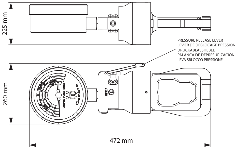
FIG. 1 MPC7 CRIMPING FORCE GAUGE DISPOSITIF MPC7 MPC7 DRUCKMESSGERÄT DISPOSITIVO MPC7 DISPOSITIVO MPC7
