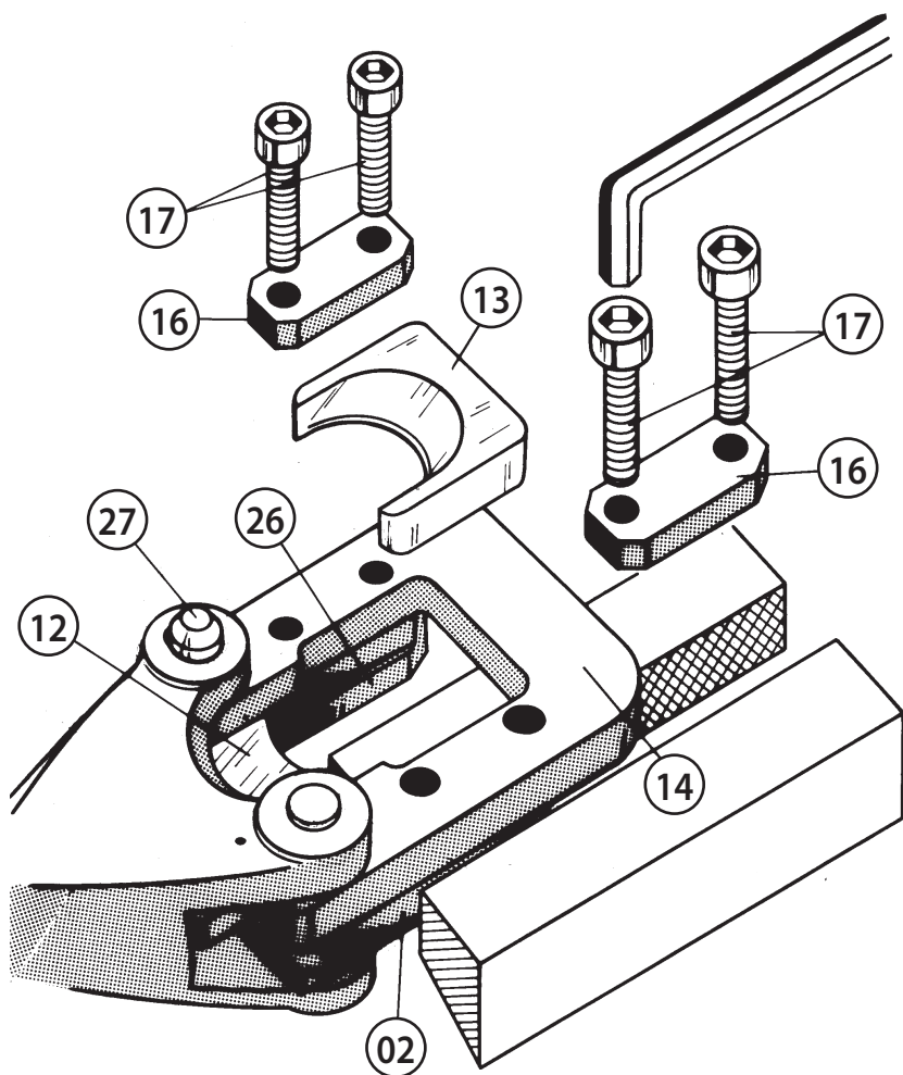
FIG. 3 UPPER BLADE REPLACEMENT CHANGEMENT LAME SUPERIEURE GEGENMESSERWECHSEL CAMBIO CUCHILLA SUPERIOR CAMBIO LAMA SUPERIORE
