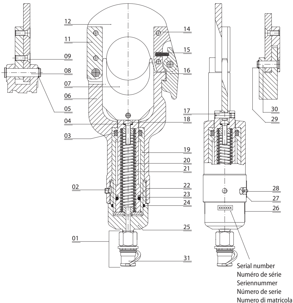
FIG. 3 LONGITUDINAL SECTION COUPE LONGITUDINALE SCHNITTZEICHNUNG SECCIÓN LONGITUDINAL SEZIONE LONGITUDINALE
