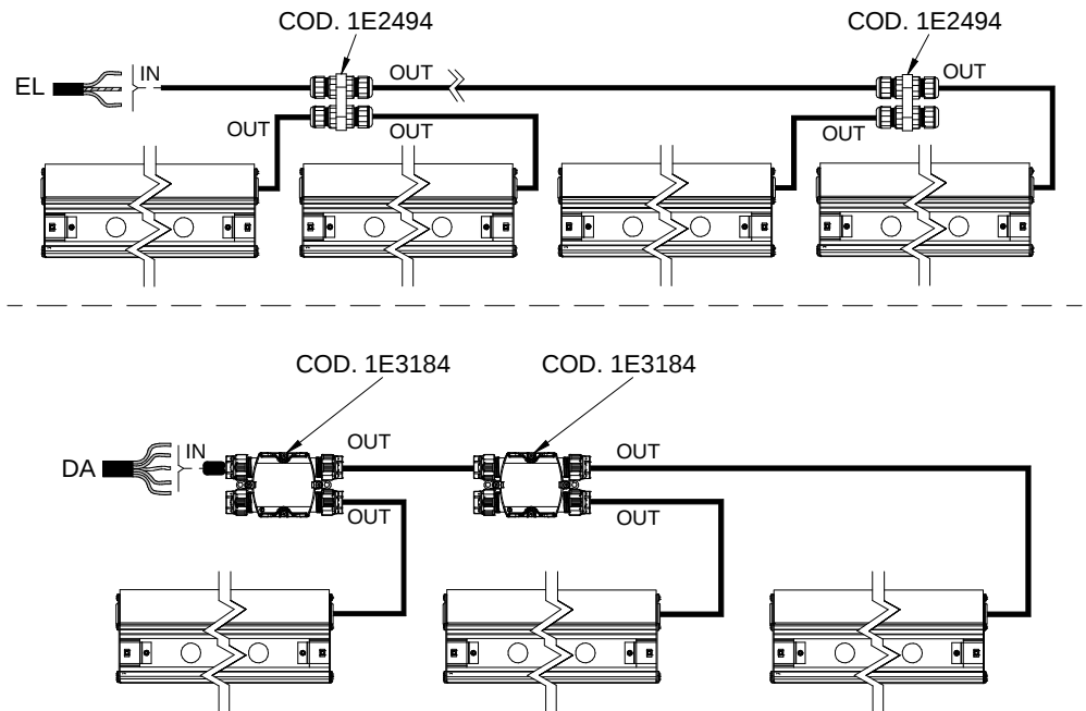
SCHEMA DI COLLEGAMENTO ALIMENTAZIONE E LOOPING WIRING SCHEME FOR MAIN AND LOOPING COLLEGAMENTO ESTERNO AL PRODOTTO / WIRING EXTERNAL PRODUCT
