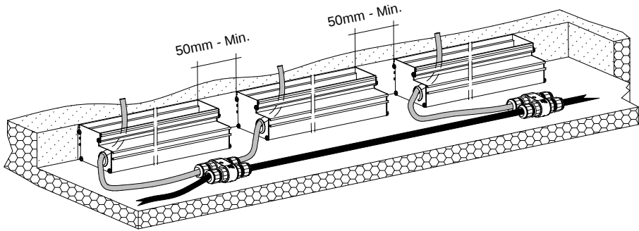
SCHEMA DI COLLEGAMENTO ALIMENTAZIONE E LOOPING WIRING SCHEME FOR MAIN AND LOOPING COLLEGAMENTO ESTERNO AL PRODOTTO / WIRING EXTERNAL PRODUCT
