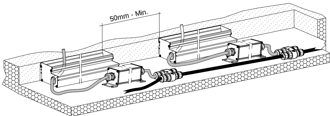
SCHEMA DI COLLEGAMENTO ALIMENTAZIONE E LOOPING WIRING SCHEME FOR MAIN AND LOOPING COLLEGAMENTO ESTERNO AL PRODOTTO / WIRING EXTERNAL PRODUCT
