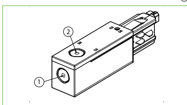
Fig. 2 Pareti sfondabili della testata Pic. 2 Knock-out walls
