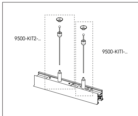
吊线组件
