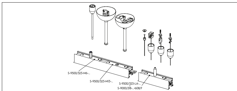
用于倒置使用轨道的配件
