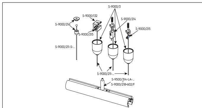
在天花板连接点有调节装置的吊线配件
