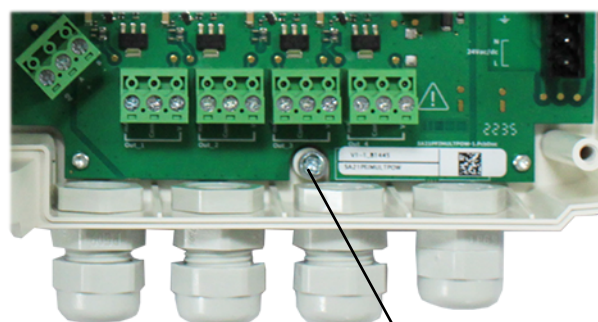
Vis de fixation du boîtier
