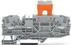
Séparateur enfiché (2006-401) dans une borne de base (2006-1661) en position ouverte
