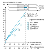
Indications pour l'utilisation des bornes à fusibles pour cartouches G Diagramme « Disposition individuelle »
