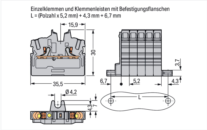
Borne de passage série 2252 avec bouton-poussoir
