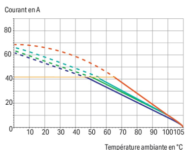
Courbe d'intensité maximale admissible Pas 7,5 mm / section de conducteur 6 mm 2 « s » Selon l'exemple de : EN 60512-5-2 / facteur de réduction 1
