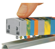
Barrette à bornes avec pieds de fixation, à monter sur rail aluminium
