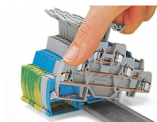
Montage d'une borne sur le rail
