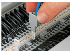
Tester avec fiche de contrôle Ici fiche de contrôle avec connexion CAGE CLAMP®
