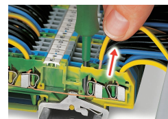
Connexion CAGE CLAMP® Déconnecter le conducteur.
