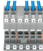
Enfichage direct des modules de fiches de contrôle dans les logements de pontage des rails conducteurs (ici série 282).
