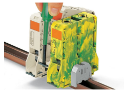
Démontage de la borne du groupe
