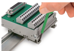
Démontage d'un module du rail.
