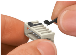
Détrompage d'un connecteur mâle - encliquer le (les) détrappeur(s)
