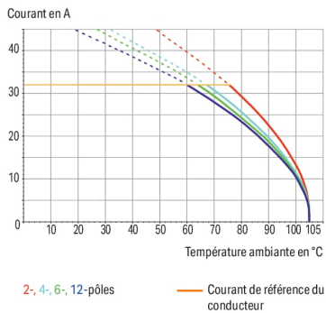
Courbe d'intensité maximale admissible Pas 5 mm / section de conducteur 4 mm² « s » Selon l'exemple de : EN 60512-5-2 / facteur de réduction 1
