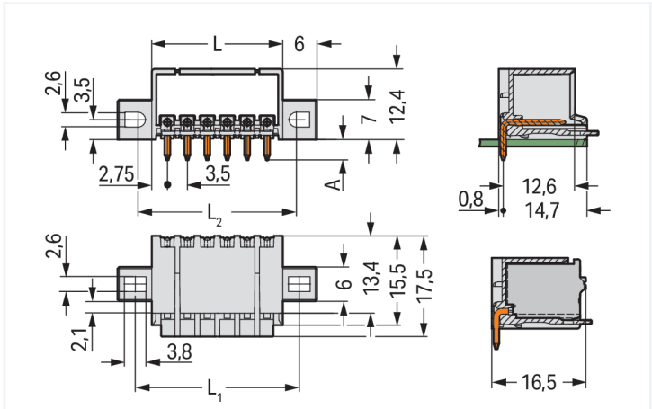
Dimensions en mm L = (nombre de pôles x pas) + 2 mm L1 = (nombre de pôles x pas) + 7,8 mm L2 = (nombre de pôles x pas) + 6,8 mm A = 3,6 mm Broche à souder THT A = 2,4 mm Broche à souder THR
