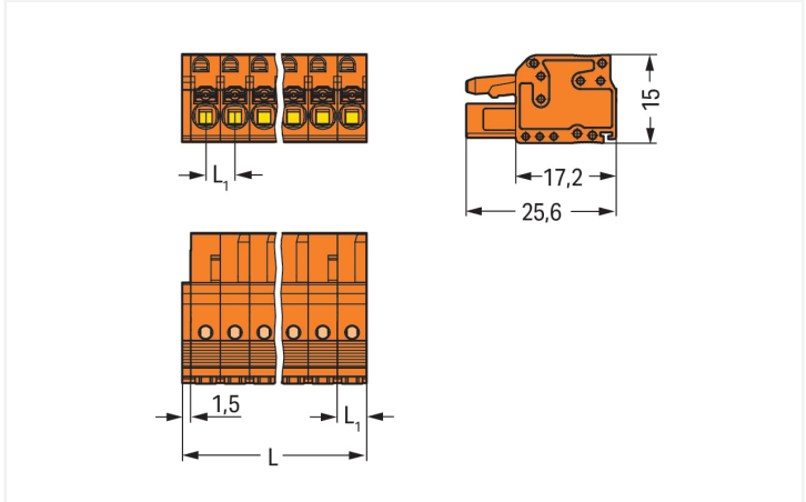
Dimensions en mm L = (\text{nombre de pôles} \times \text{pas}) + 1,5 \text{ mm} L1 = 5,08 \text{ mm} Connecteurs femelles de 2 à 3 pôles – seulement 1 crochet d'arrêt
