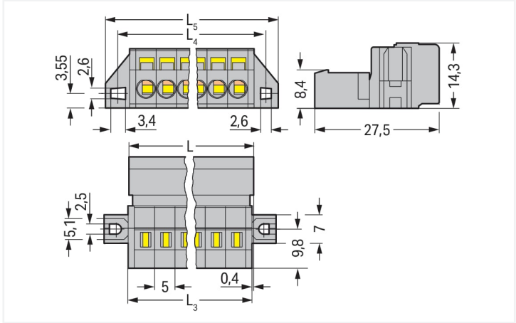
Dimensions en mm L = (Nombre de pôles – 1) x pas + 8,2 mm L3 = L – 0,2 mm L4 = L3 + 5,8 mm L5 = L3 + 11,8 mm
