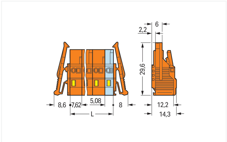
Dimensions en mm L = (nombre pôles – 1) x pas + 5,08 mm Connecteurs femelles de 2 à 3 pôles – seulement 1 crochet d'arrêt
