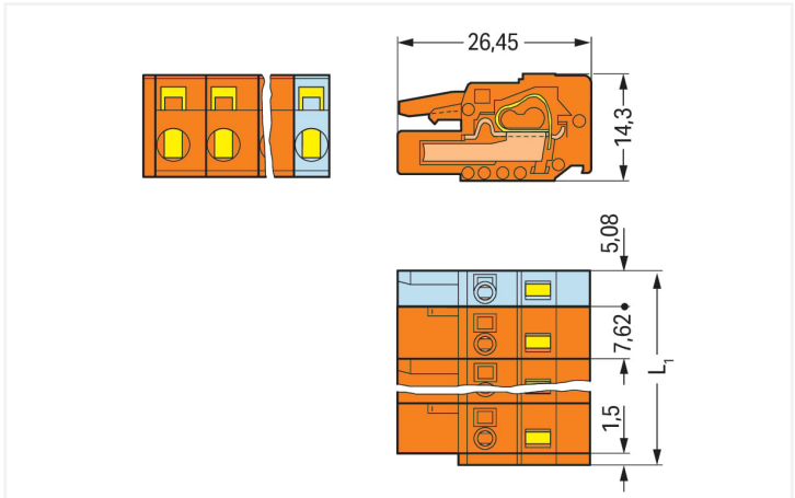
Dimensions en mm L1 = (\text{Nombre de pôles} - 1) \times \text{pas} + 5,08 \text{ mm} + 1,5 \text{ mm} Connecteurs femelles de 2 à 3 pôles – seulement 1 crochet d'arrêt
