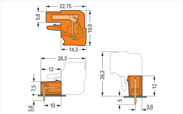
Dimensions en mm Longueur totale = (nombre de pôles x pas) + 1,5 mm + 0,9 mm Connecteurs femelles de 2 à 3 pôles – seulement 1 crochet d'arrêt
