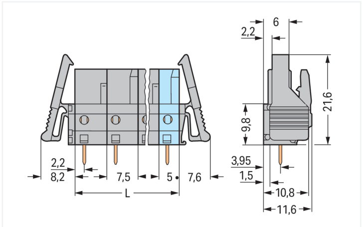
Dimensions en mm L = (\text{Nombre de pôles} - 1) \times \text{pas} + 5 \text{ mm} Connecteurs femelles de 2 à 3 pôles – seulement 1 crochet d'arrêt
