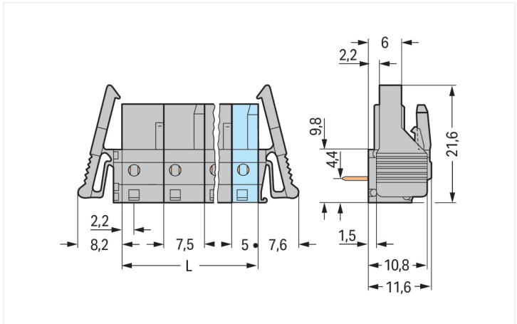
Dimensions en mm L = (Nombre de pôles – 1) x pas + 5 mm Distance à la première broche à souder 2,2 mm Connecteurs femelles de 2 à 3 pôles – seulement 1 crochet d'arrêt
