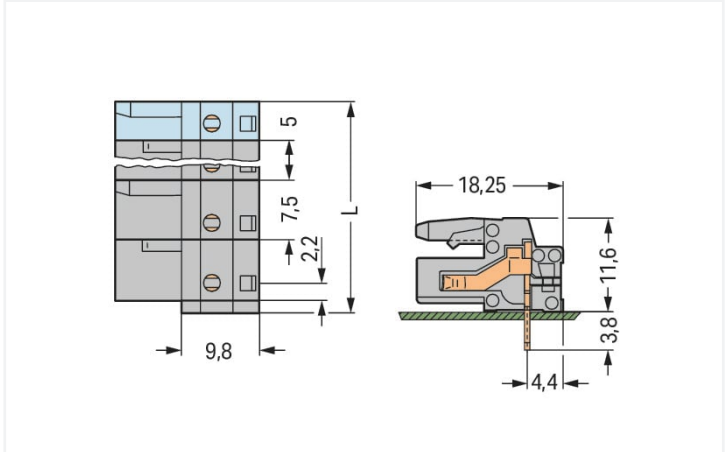
Dimensions en mm L = (\text{nombre de pôles} - 1) \times \text{pas} + 5 \text{ mm} + 1,5 \text{ mm} Connecteurs femelles de 2 à 3 pôles – seulement 1 crochet d'arrêt
