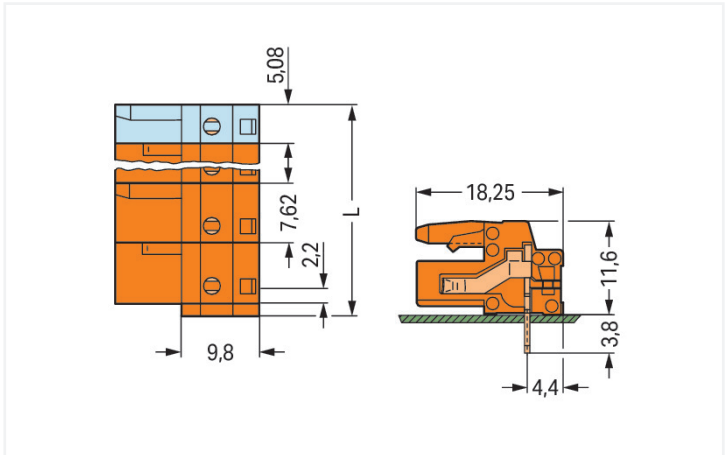
Dimensions en mm L = (nombre de pôles - 1) x pas + 5,08 mm + 1,5 mm Connecteurs femelles de 2 à 3 pôles – seulement 1 crochet d'arrêt
