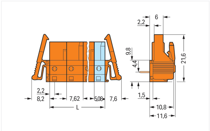
Dimensions en mm L = (nombre pôles – 1) x pas + 5,08 mm Distance à la première broche à souder 2,2 mm Connecteurs femelles de 2 à 3 pôles – seulement 1 crochet d'arrêt
